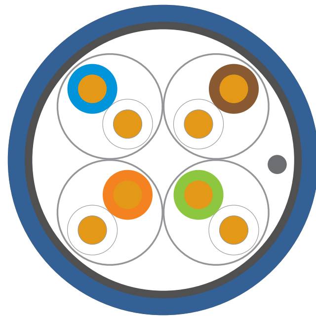
F/FTP
