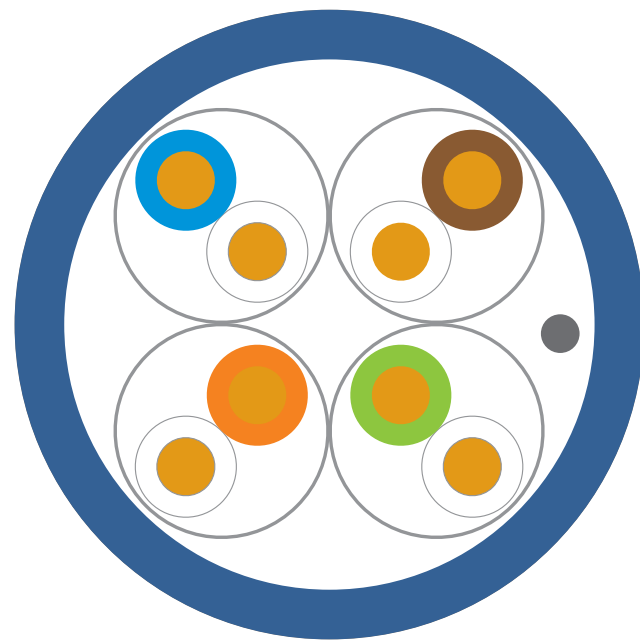
U/FTP
