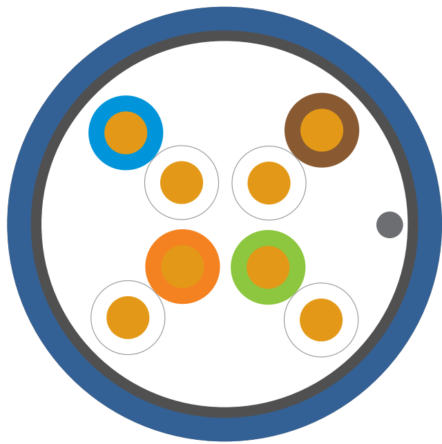
F/UTP
